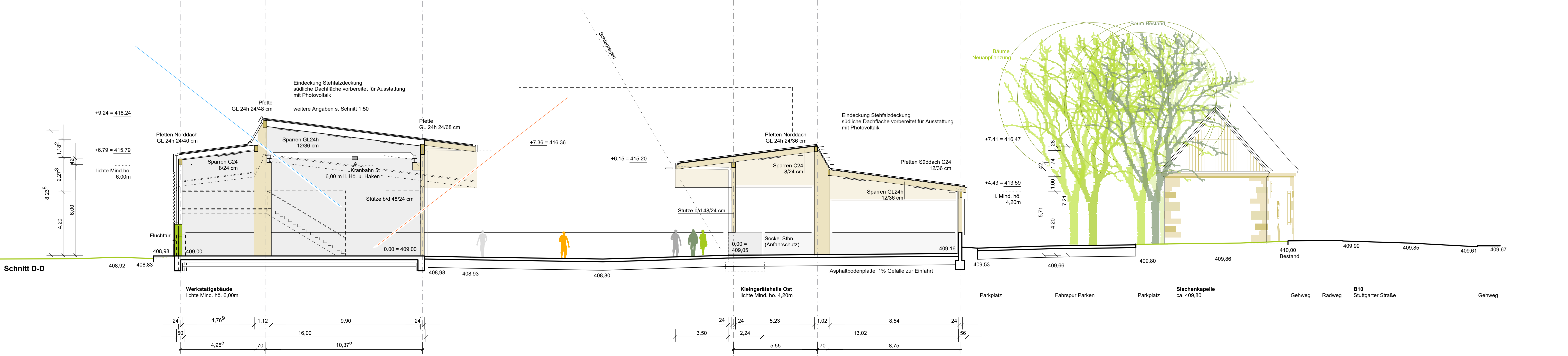
Schnitt D-D
